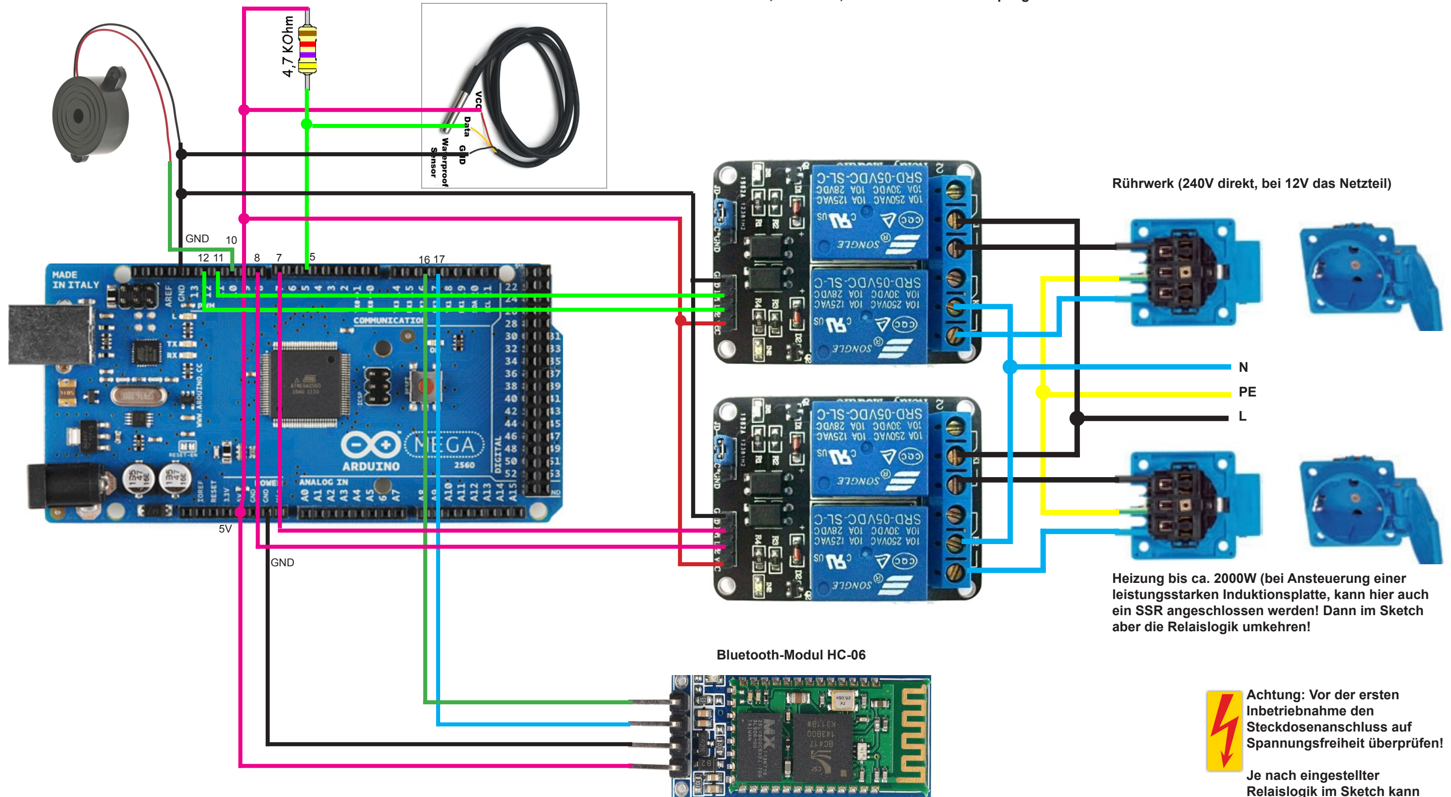
DS18B20- Temperatursensor
